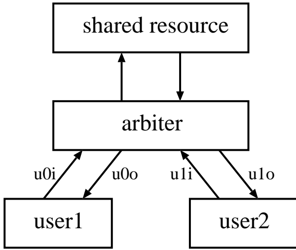
Fig. 2. An arbiter module.
