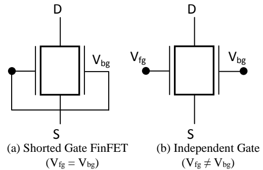
Fig. 1 FinFET Models
